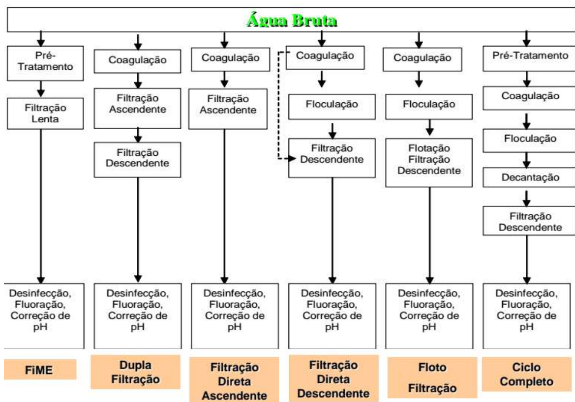
FIGURA 6 - ESQUEMATIZAÇÃO DOS TIPOS MAIS COMUNS DE TRATAMENTO DE ÁGUA.
