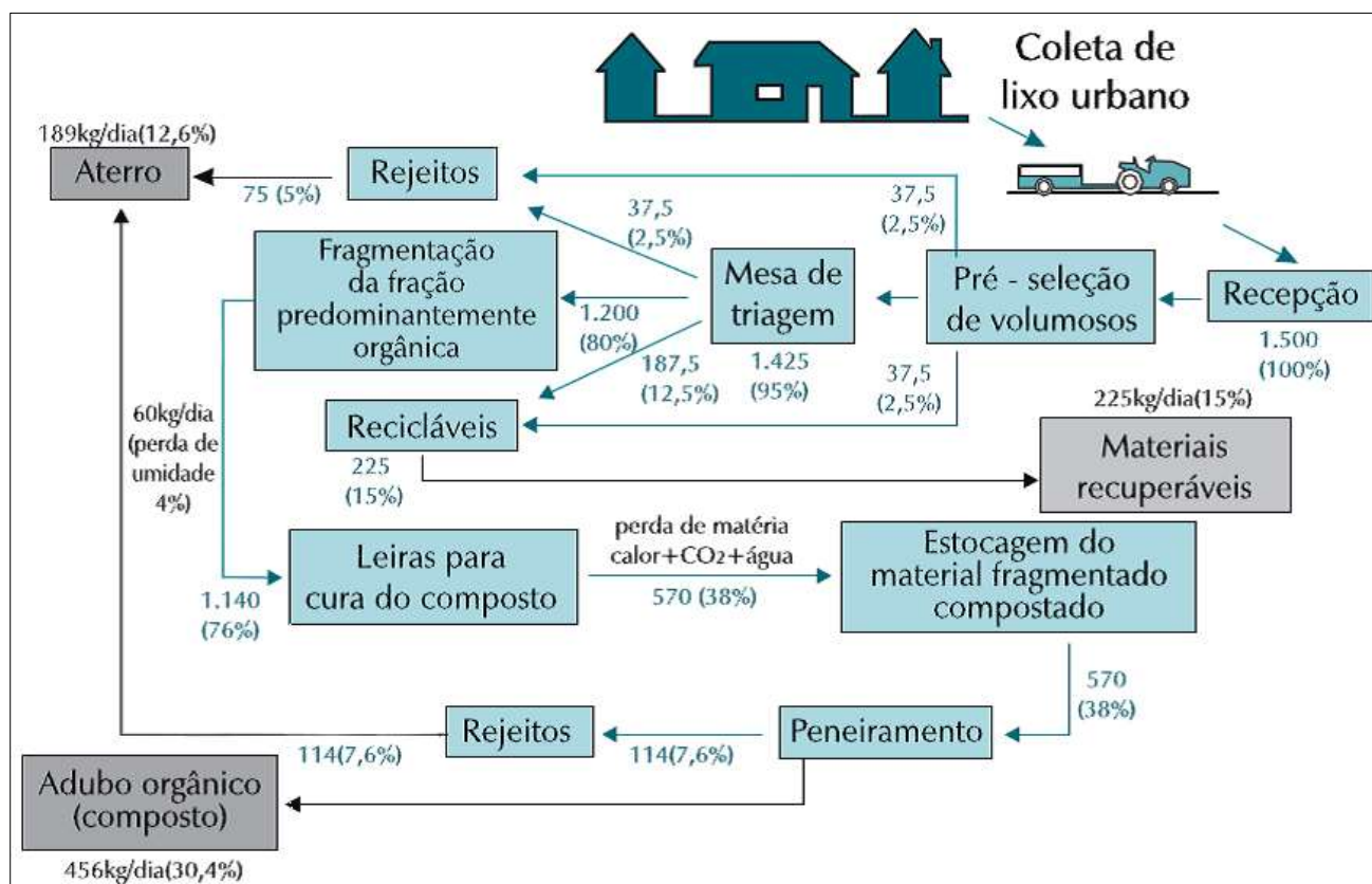
FIGURA 14 - USINA DE TRIAGEM E COMPOSTAGEM.
