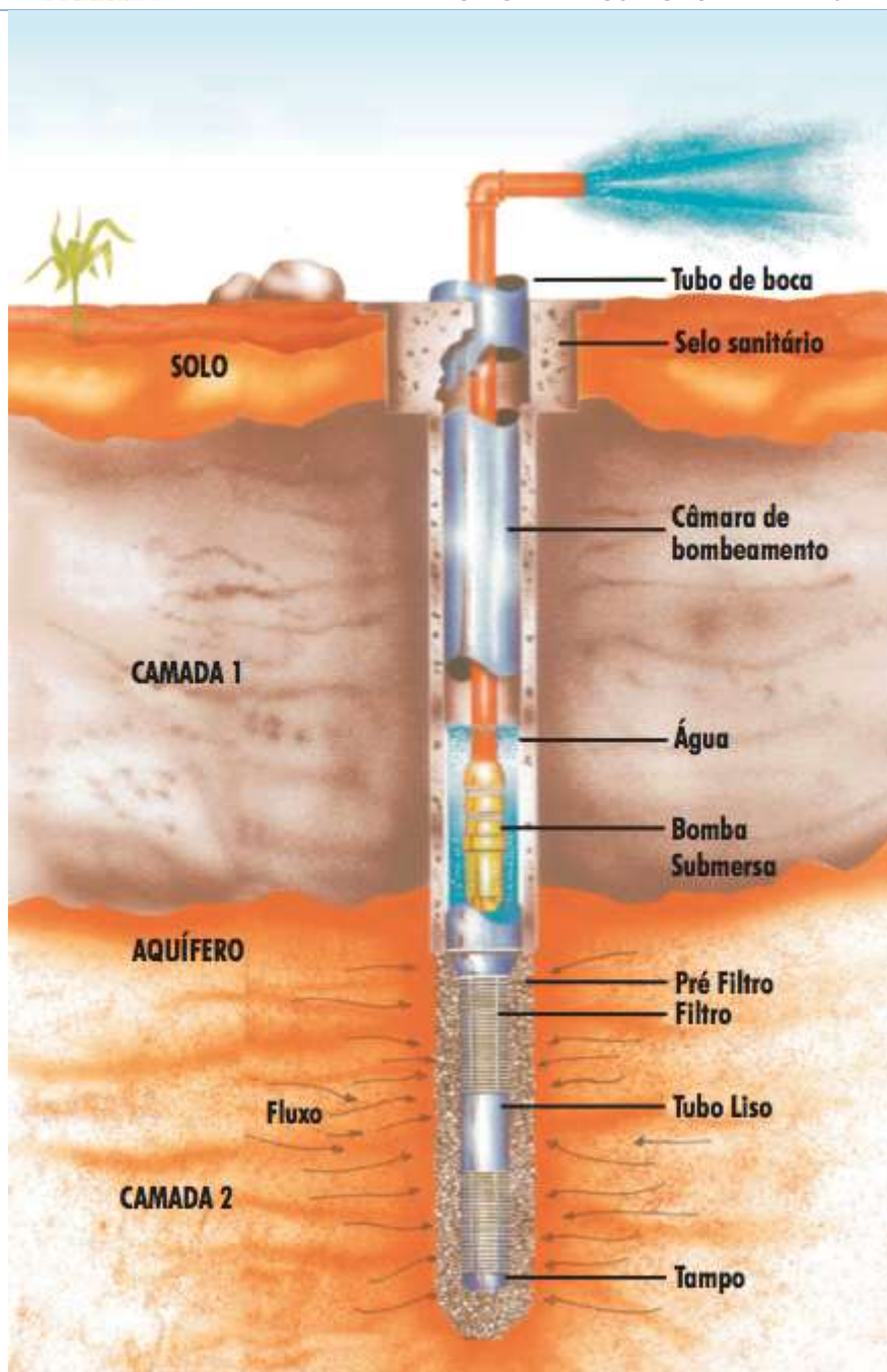
FIGURA 4 - ESQUEMATIZAÇÃO DE UM POÇO PROFUNDO.
