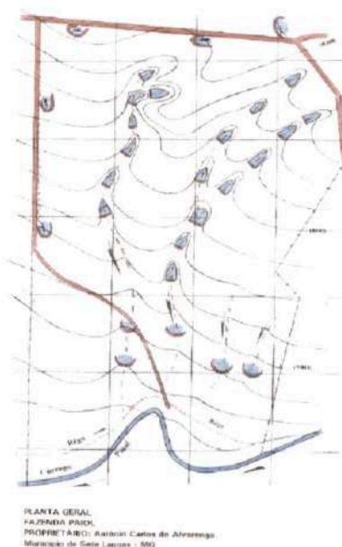
IMAGEM 23: Orientação e tipologia para a construção de barraginhas. (Barros, 1998).
