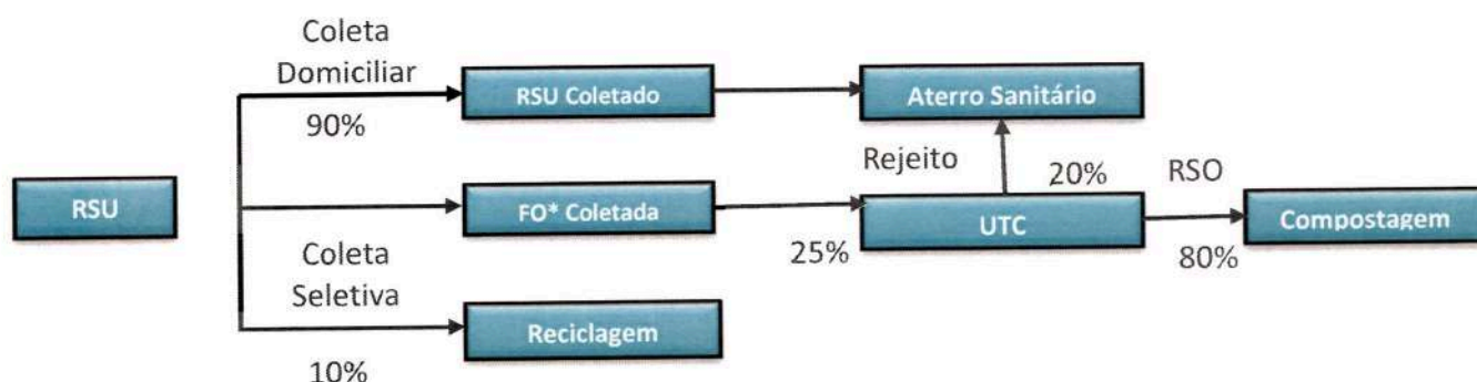
IMAGEM 05: Esquema do Cenário 4-1: com coleta seletiva e UC. Opção 1: 25% dos RSO são encaminhados para compostagem na UC. (RSU = RSD)
