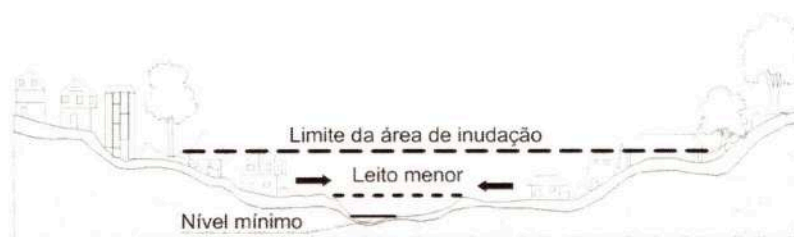
IMAGEM 17: Características do leito dos rios.
