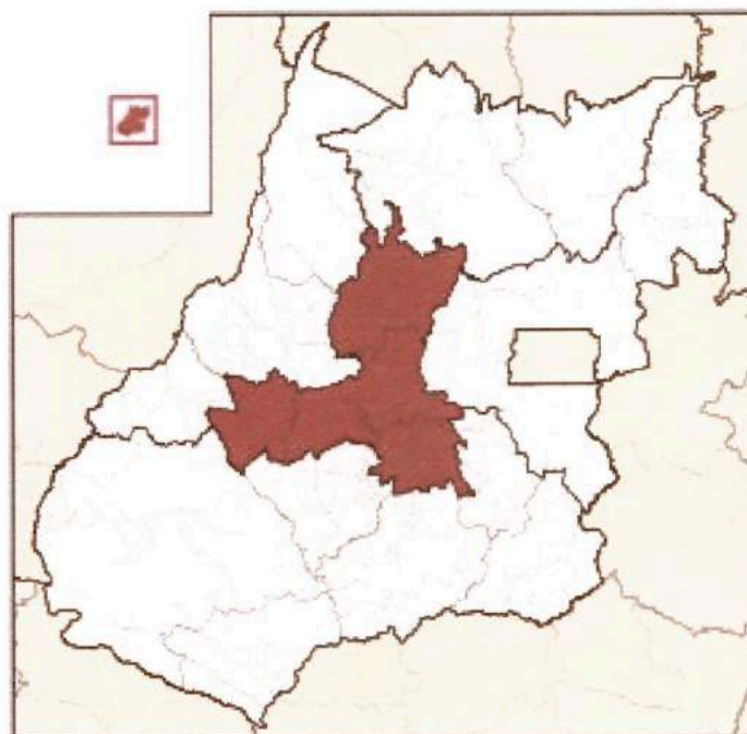
IMAGEM 03: Localização da mesorregião Centro Goiano.
