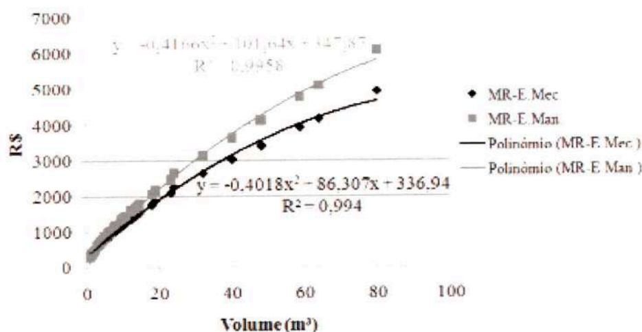
IMAGEM 07: Gráfico da variação dos custos totais dos microreservatórios por volume controlado (Francisco, 2010).
