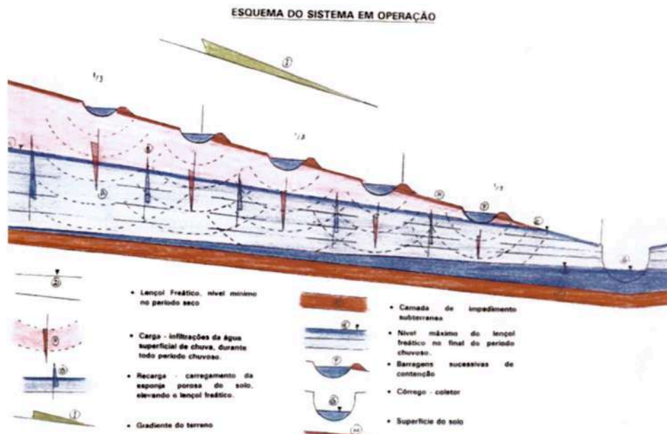
IMAGEM 24: Esquema do sistema de operação de barraginhas. (Barros, 1998).
