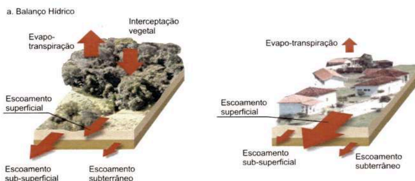
IMAGEM 18: Alterações dos fluxos do balanço hídrico causado pela urbanização.
