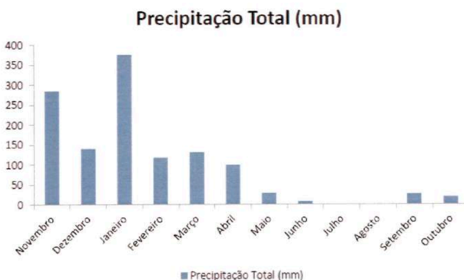
IMAGEM 08: Gráfico da precipitação total - novembro de 2012 à outubro de 2013.
